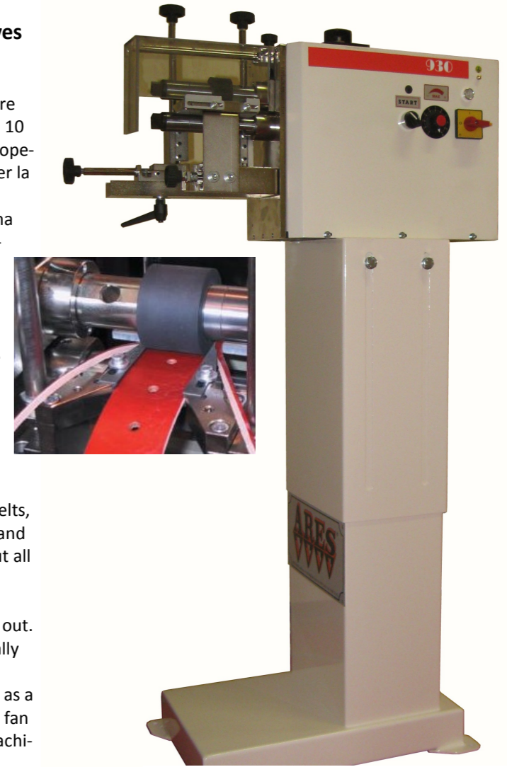
930 con appoggio optional ad altezza regolabile 930 with optional adjustable height base
